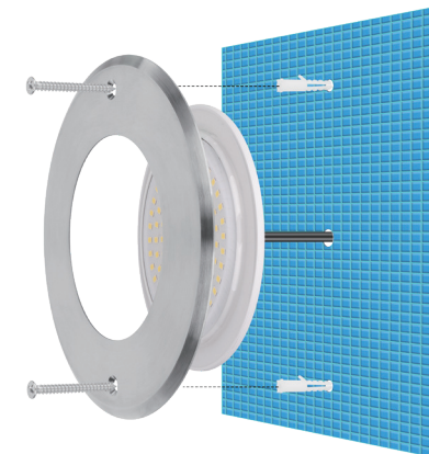
安装指引图 (Installation guide drawing)
