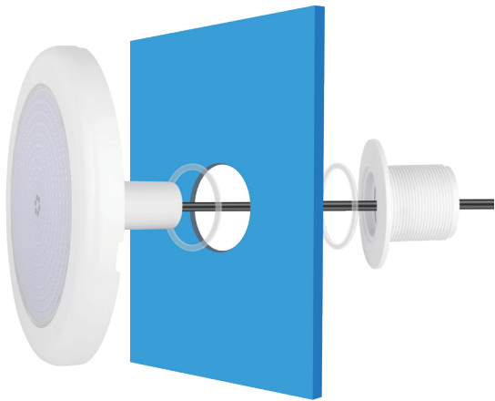
安装指引图 (Installation guide drawing)
