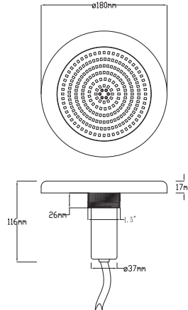
产品尺寸 (Product size)
