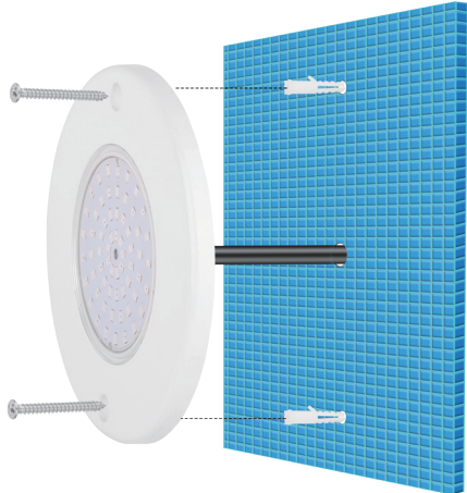
安装指引图 (Installation guide drawing)
