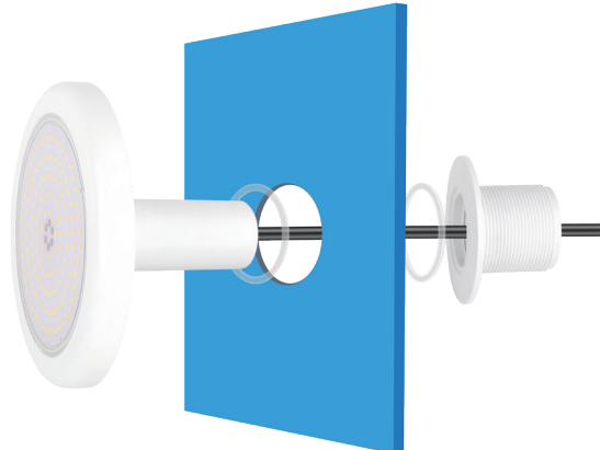
安装指引图 (Installation guide drawing)
