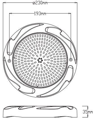
产品尺寸 (Product size)
