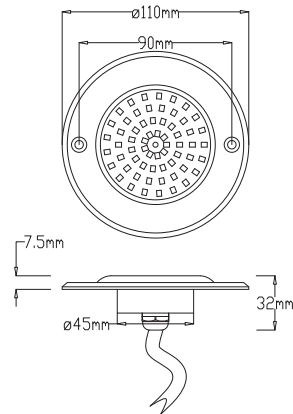
产品尺寸 (Product size)
