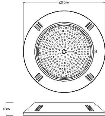
产品尺寸 (Product size)
