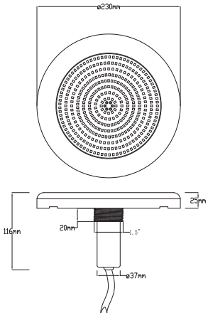
产品尺寸 (Product size)
