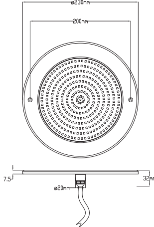
产品尺寸 (Product size)
