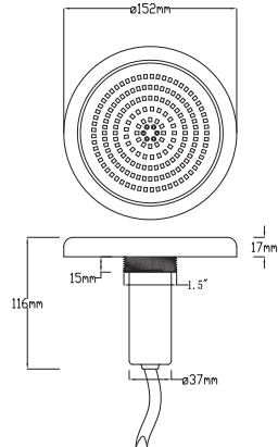
产品尺寸 (Product size)
