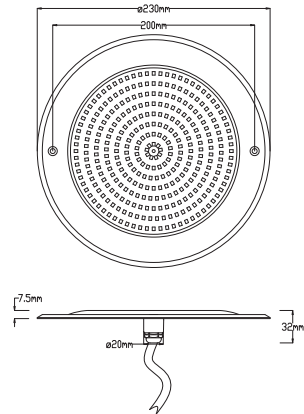
产品尺寸 (Product size)
