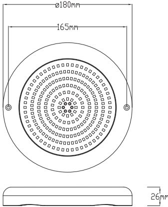
产品尺寸 (Product size)
