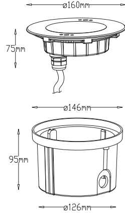
产品尺寸 (Product size)
