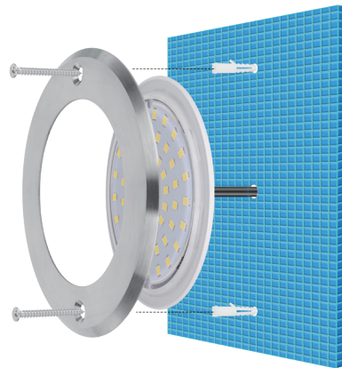
安装指引图 (Installation guide drawing)
