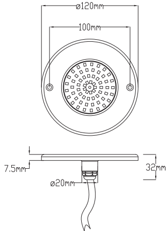
产品尺寸 (Product size)
